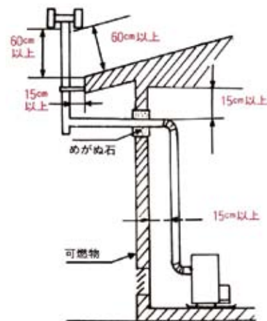
〈煙突の設置〉
